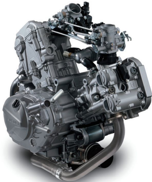
Motor DOHC V-Twin a 90° de 645 cc
